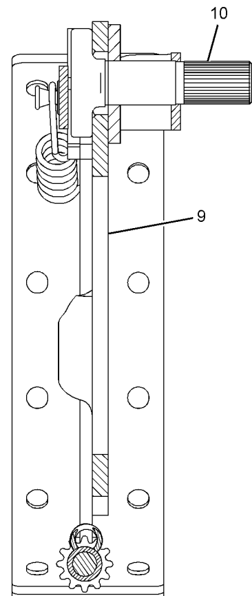
SECTION A-A
