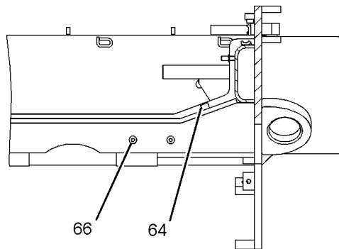
SECTION D-D
