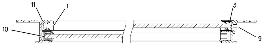
SECTION A-A
