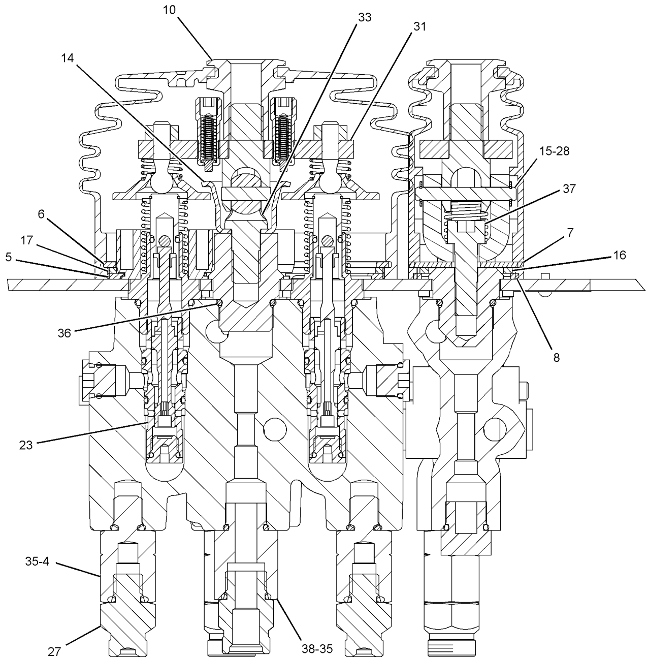
SECTION D-D
