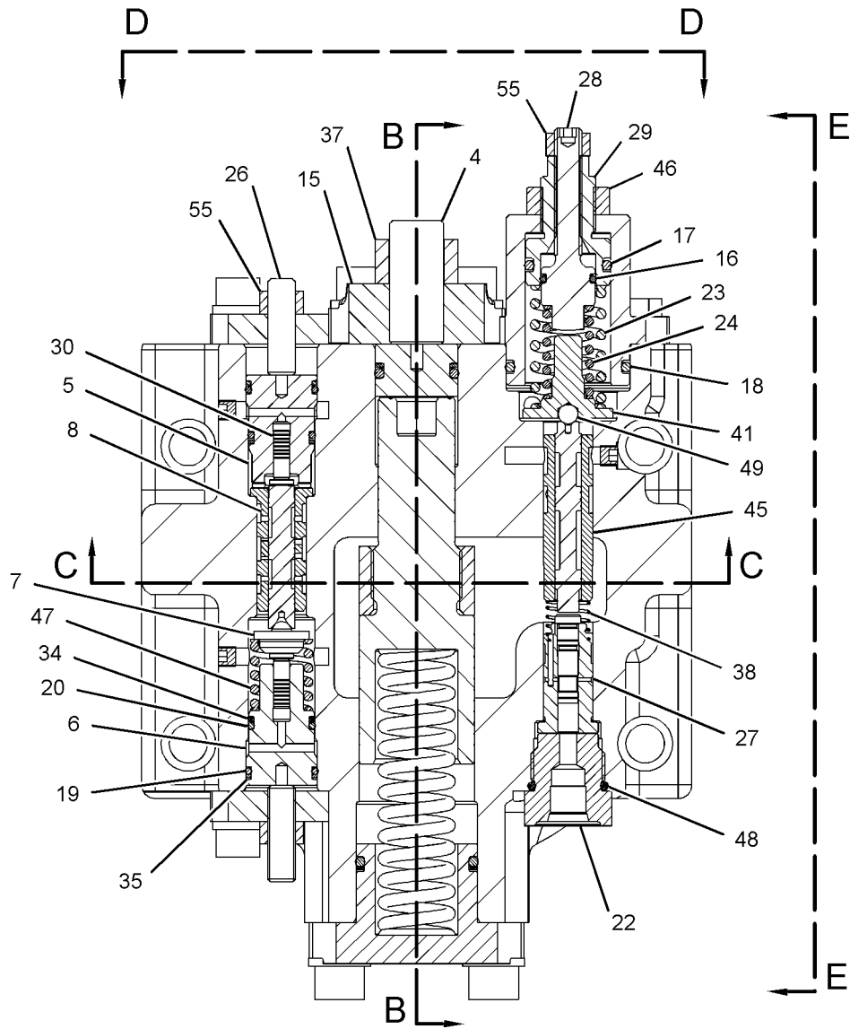
SECTION A-A
