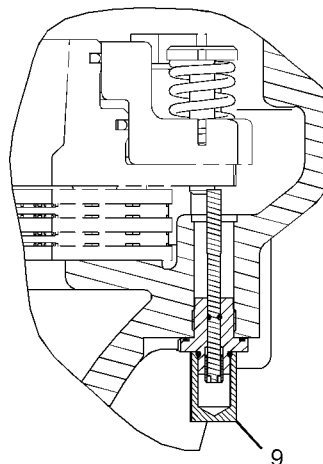
SECTION D-D
