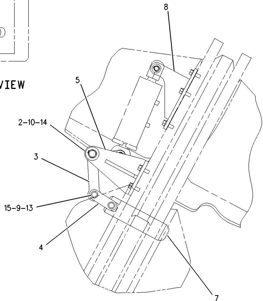
VIEW A-A
