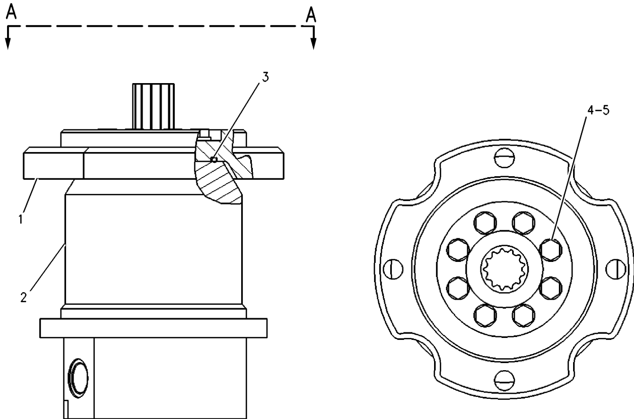
VIEW A-A
