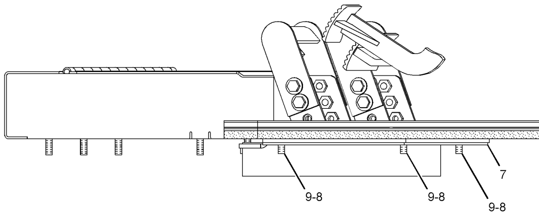
VIEW A-A
