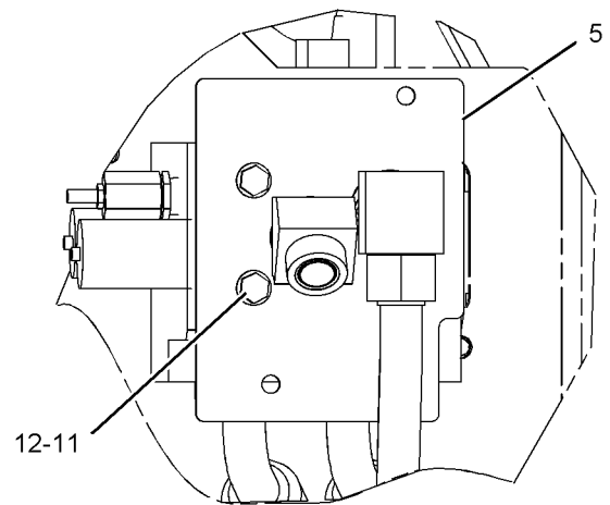
VIEW A-A
