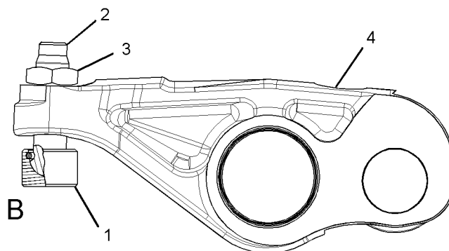
VIEW A-A
