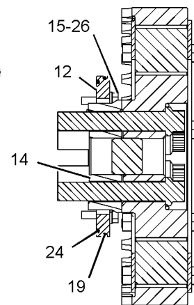
SECTION D-D
