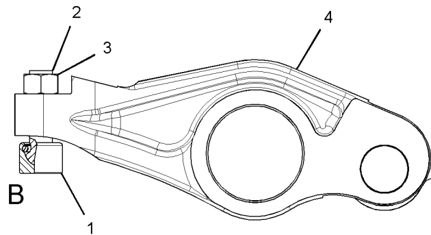
VIEW A-A
