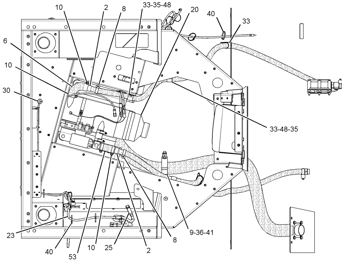
VIEW A-A
