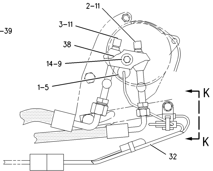
VIEW A-A
