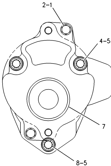
VIEW A-A
