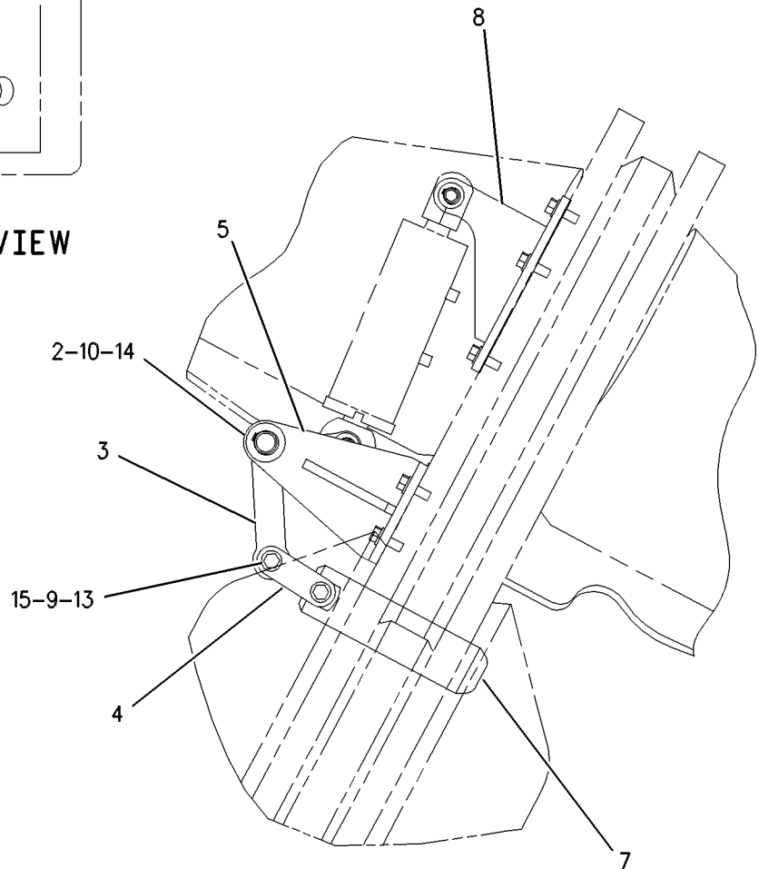
VIEW A-A
