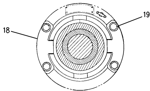
VIEW A-A
