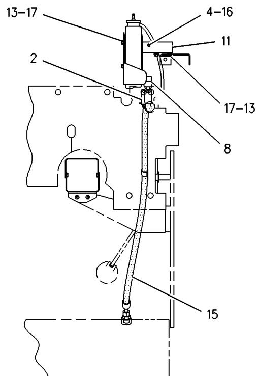
VIEW A-A
