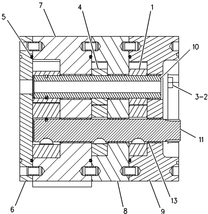
SECTION A-A
