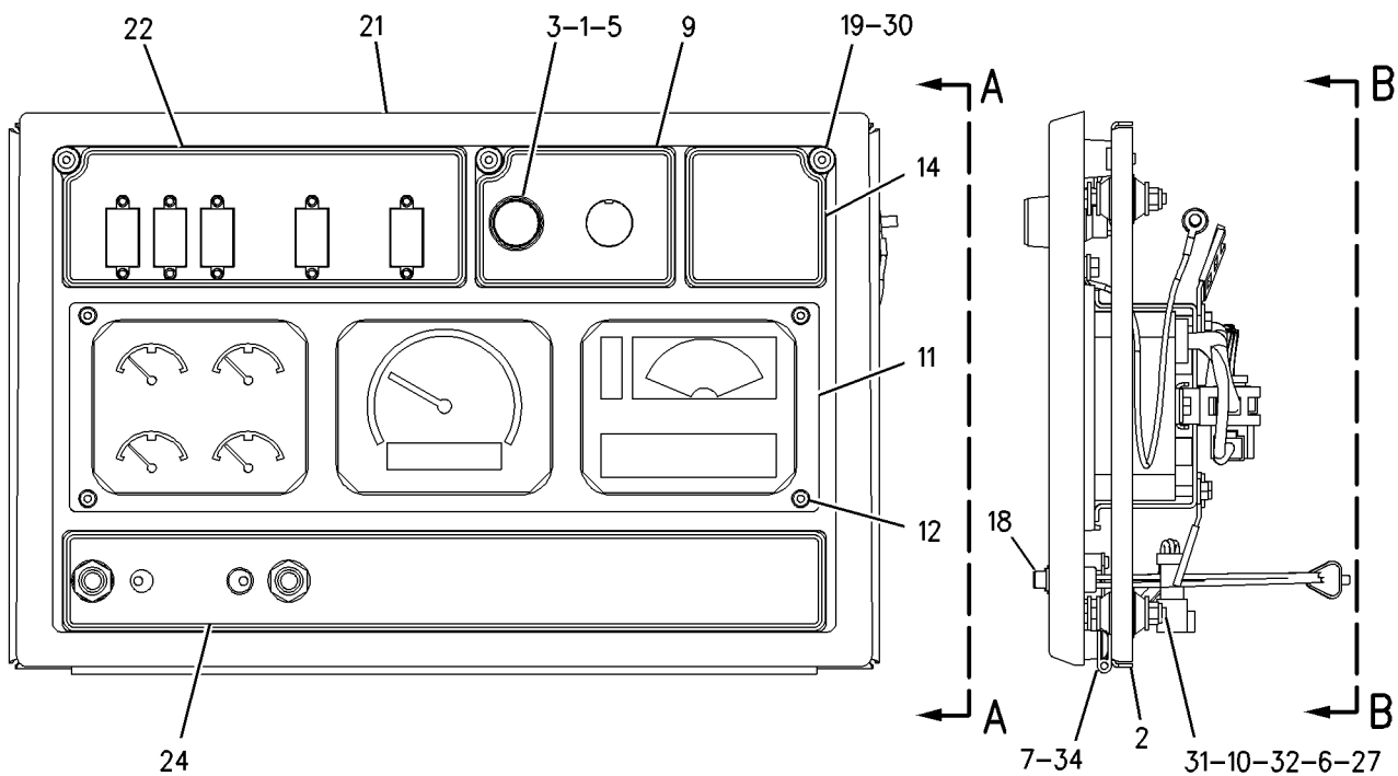
VIEW A-A
