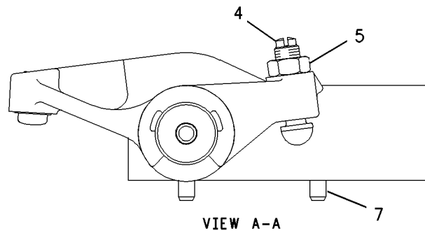
VIEW A-A
