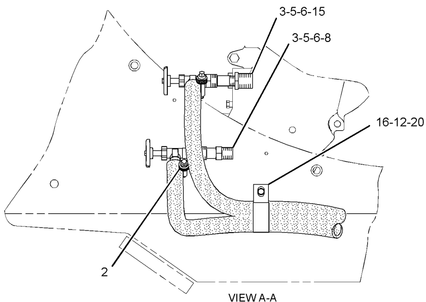
VIEW A-A
