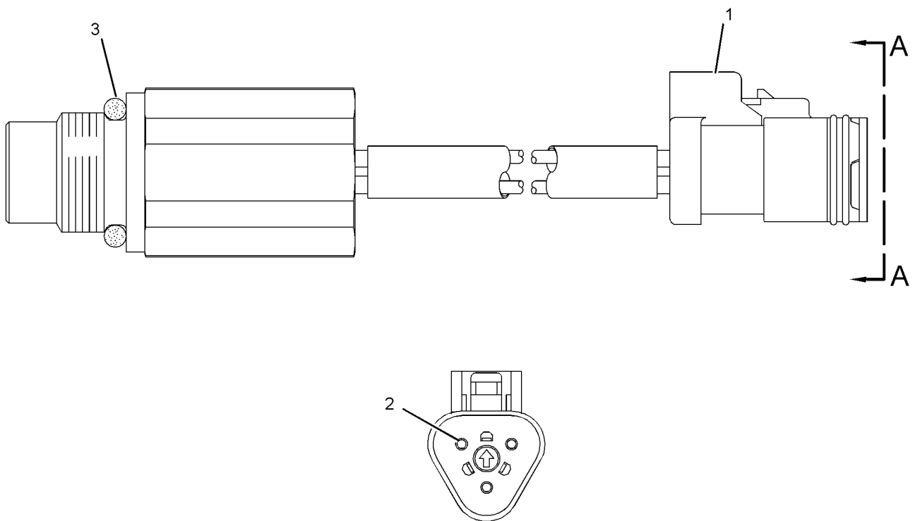
VIEW A-A
