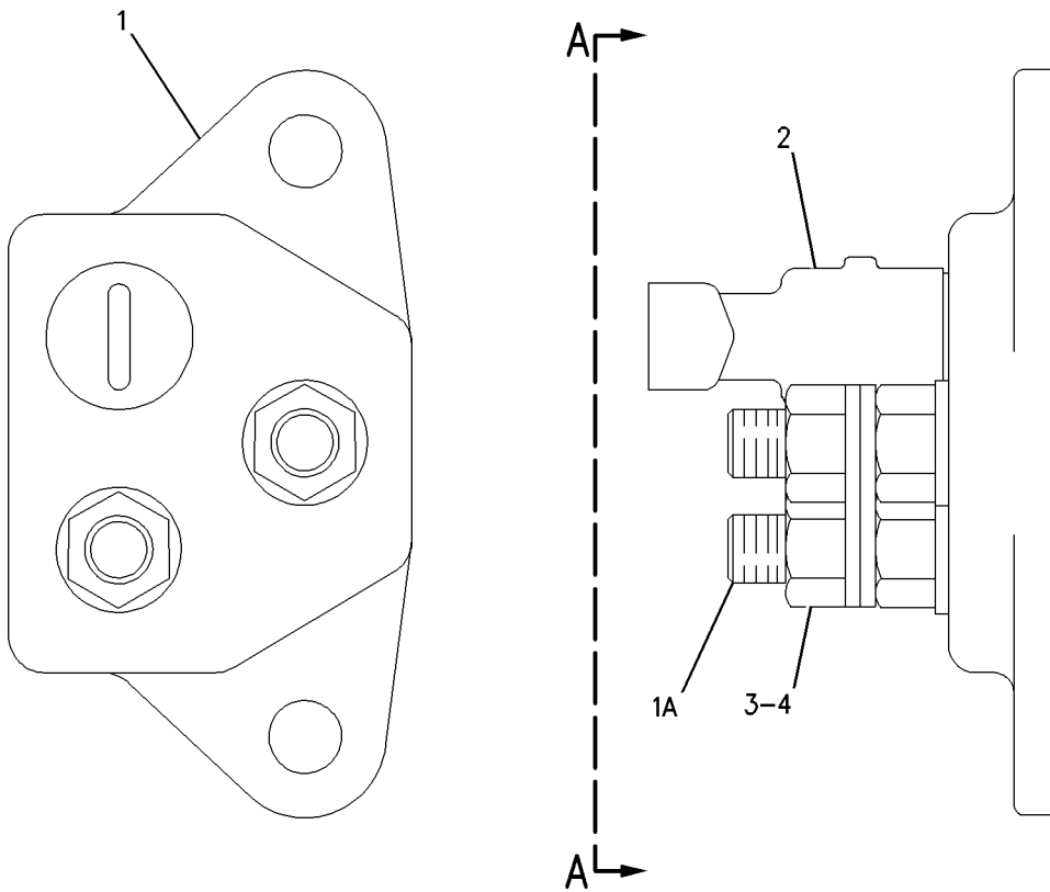
VIEW A-A
