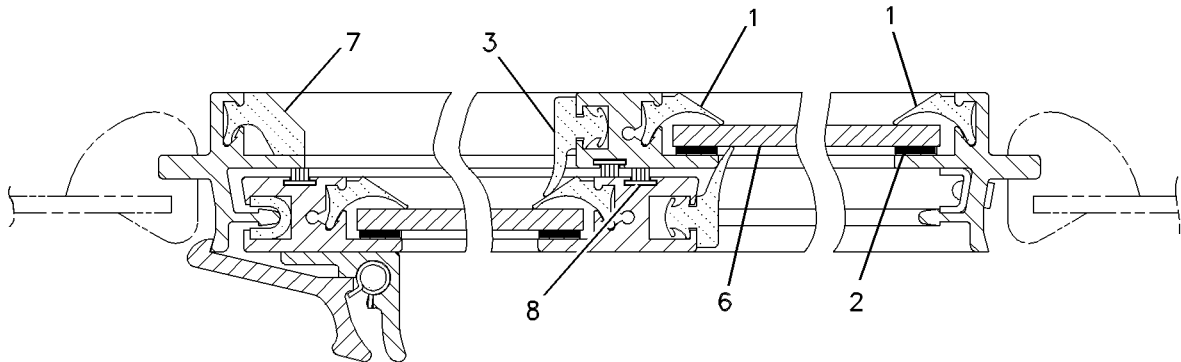
SECTION A-A
