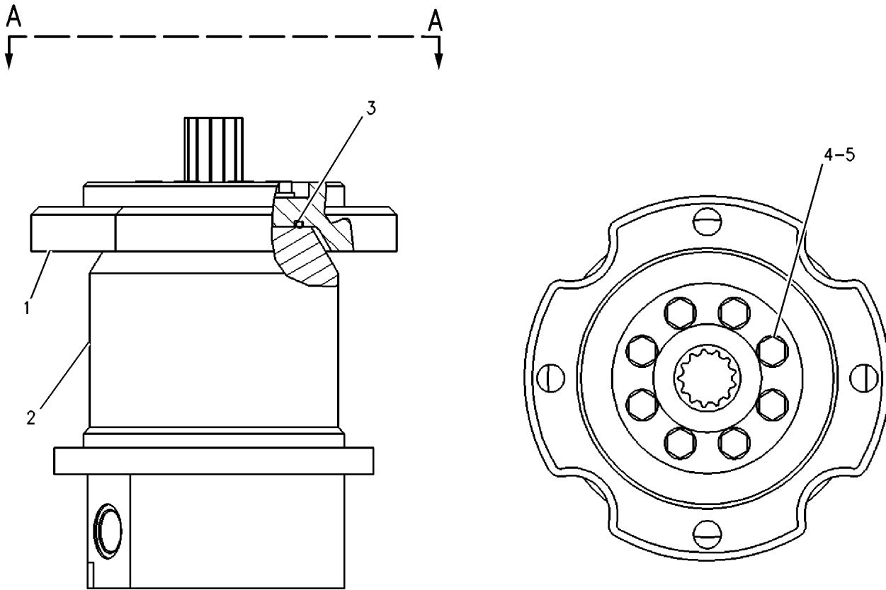
VIEW A-A
