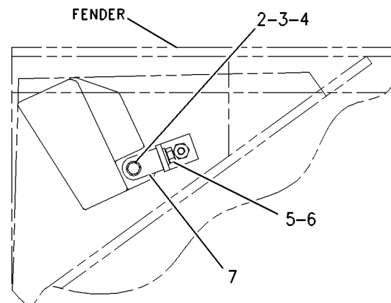
VIEW A-A
