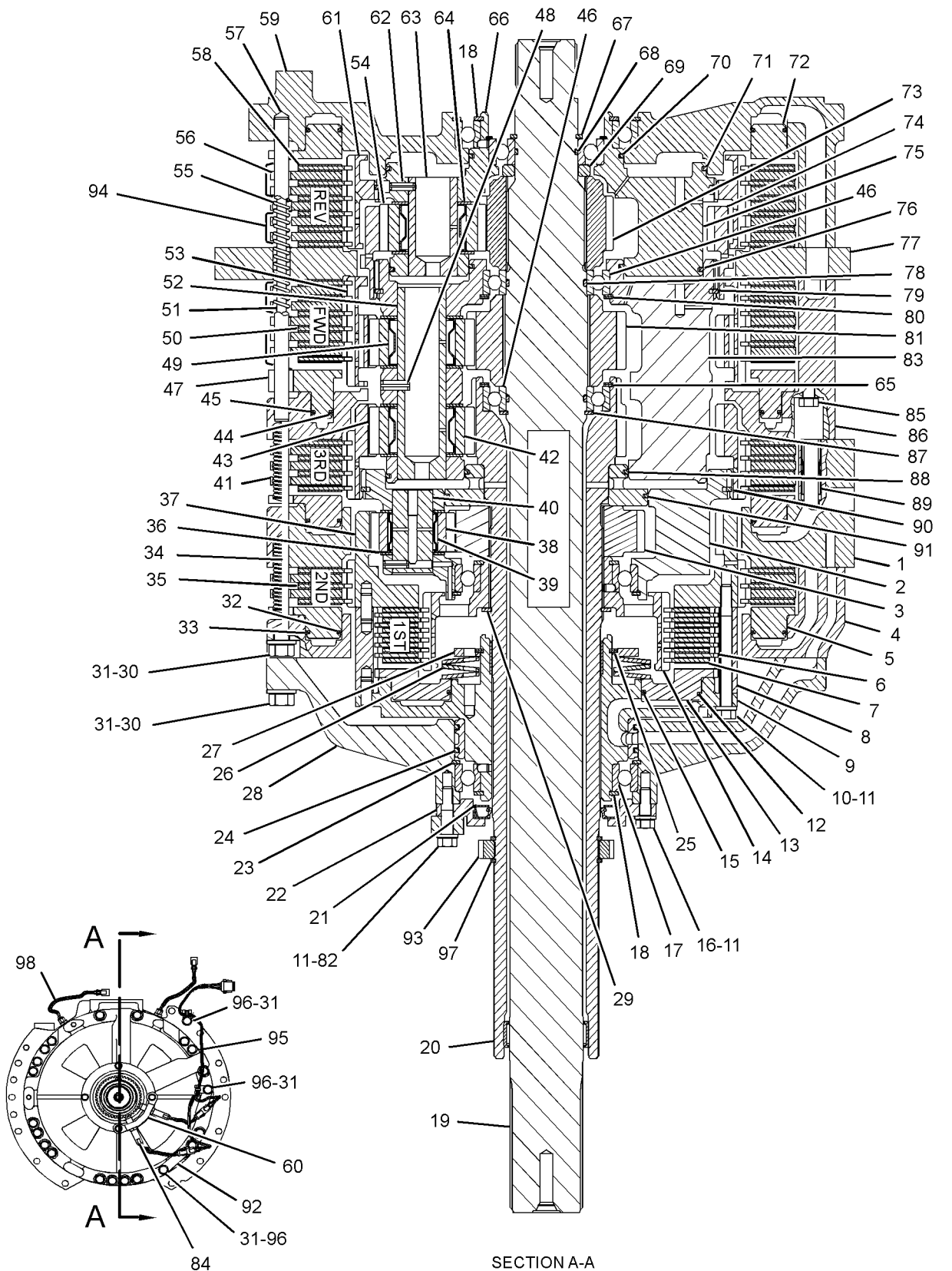
SECTION A-A
