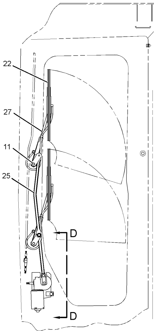
LH DOOR
