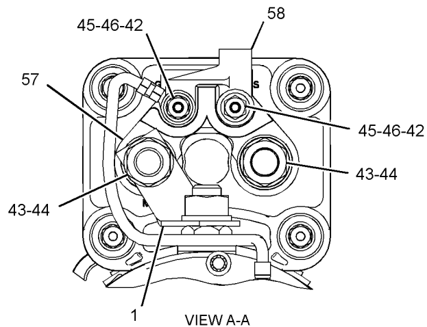
VIEW A-A
