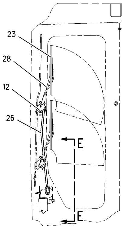
LH DOOR
