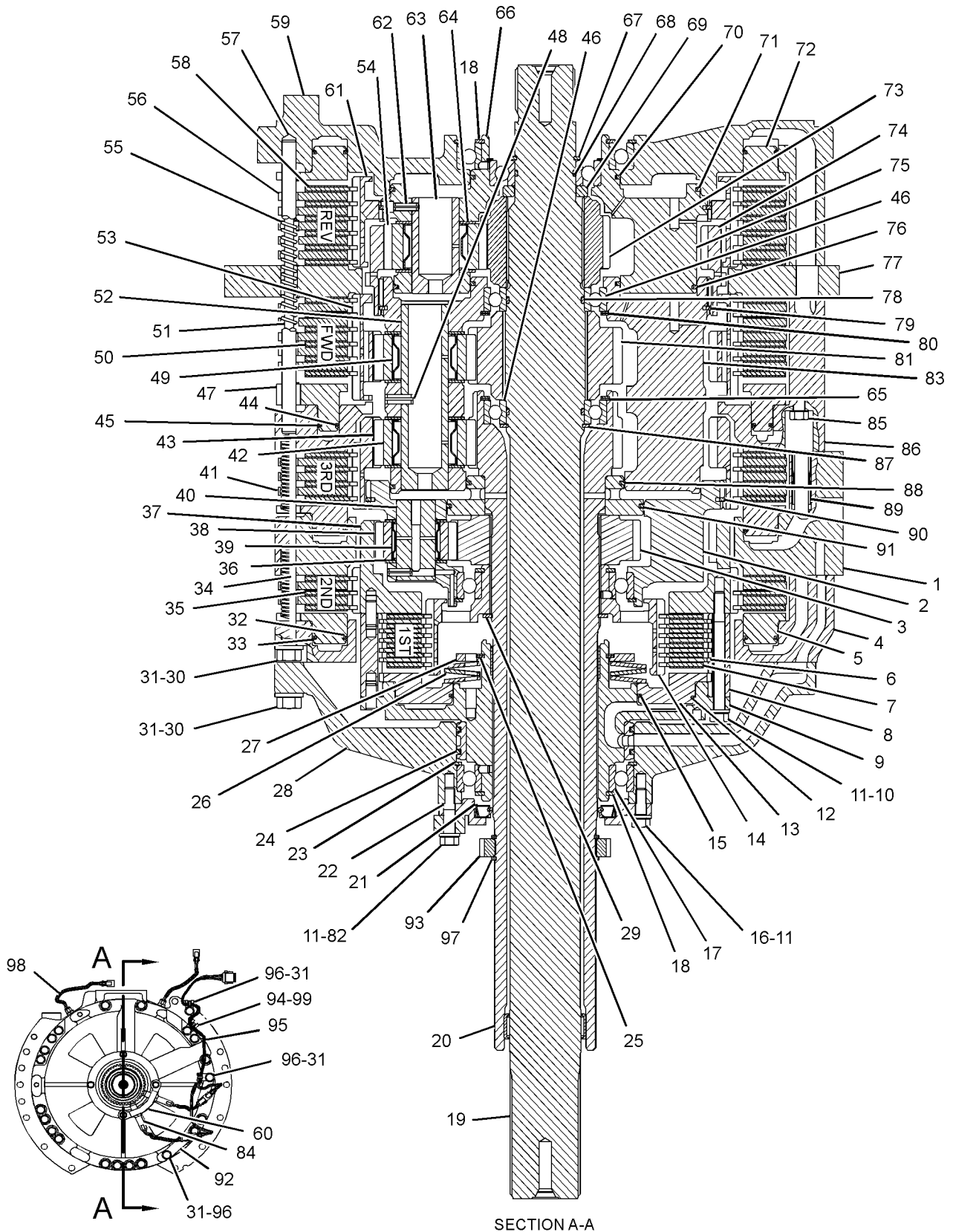
SECTION A-A
