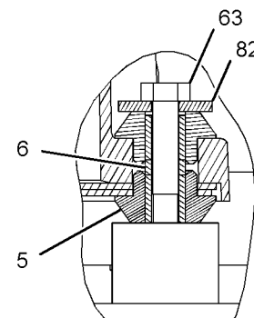
SECTION V-V
