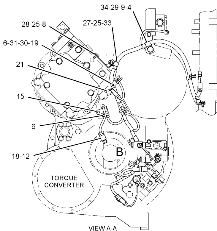
VIEW A-A
