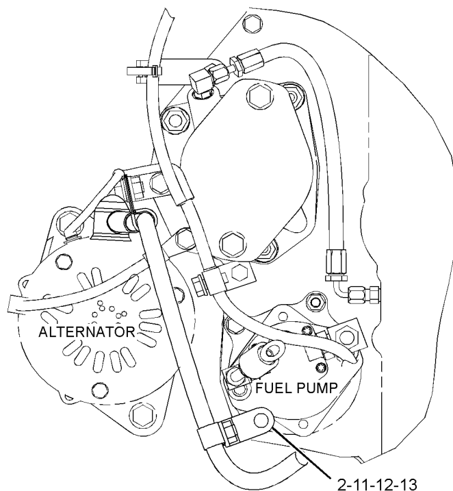
VIEW A-A
