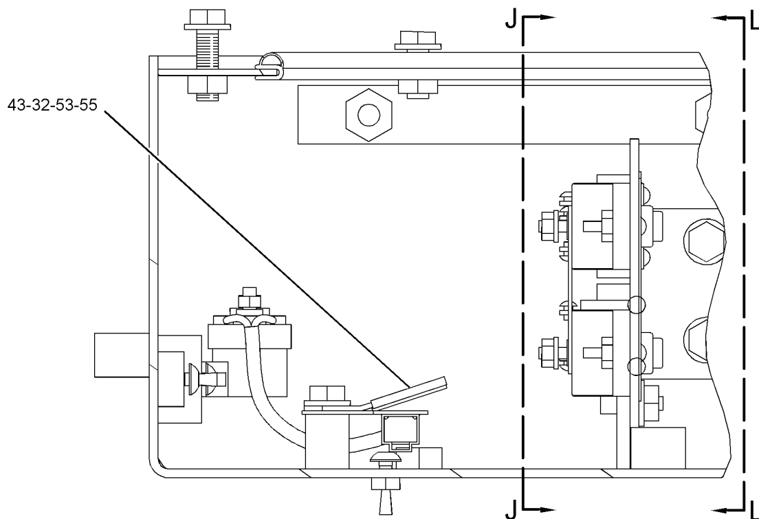
SECTION D-D
