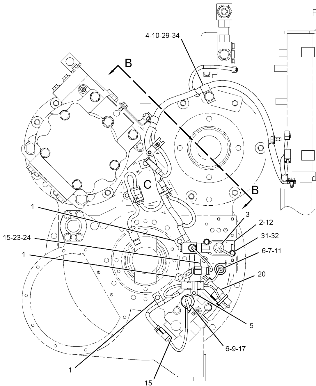
VIEW A-A
