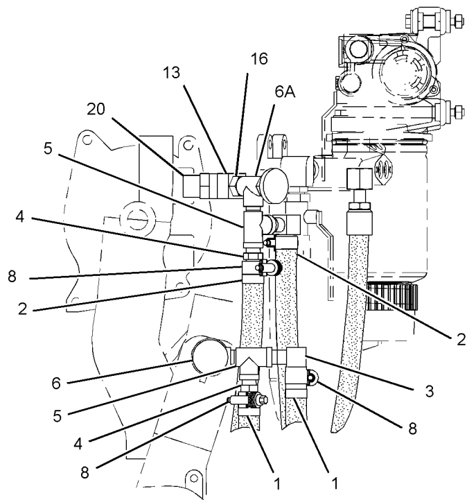
VIEW A-A
