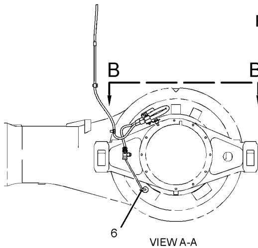
VIEW A-A
