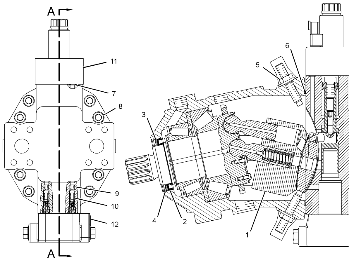
SECTION A-A
