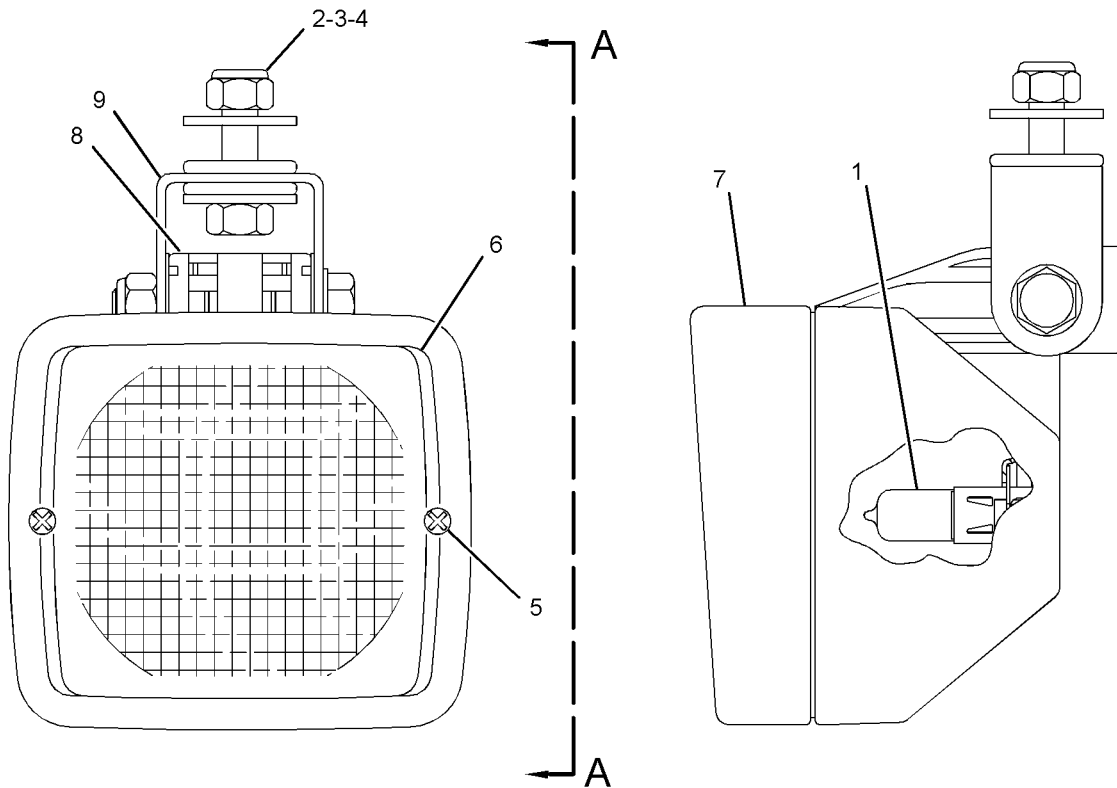
VIEW A-A
